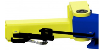
Dispositif de retenue des bras de levage pivotants automatique
