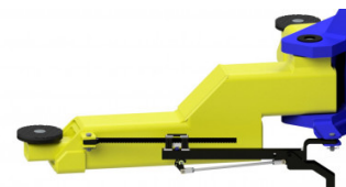
Dispositif de retenue des bras de levage pivotants automatique
