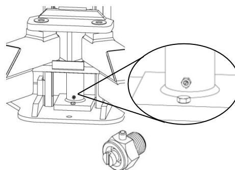
FIGURE 12 : PURGEUR D'AIR
