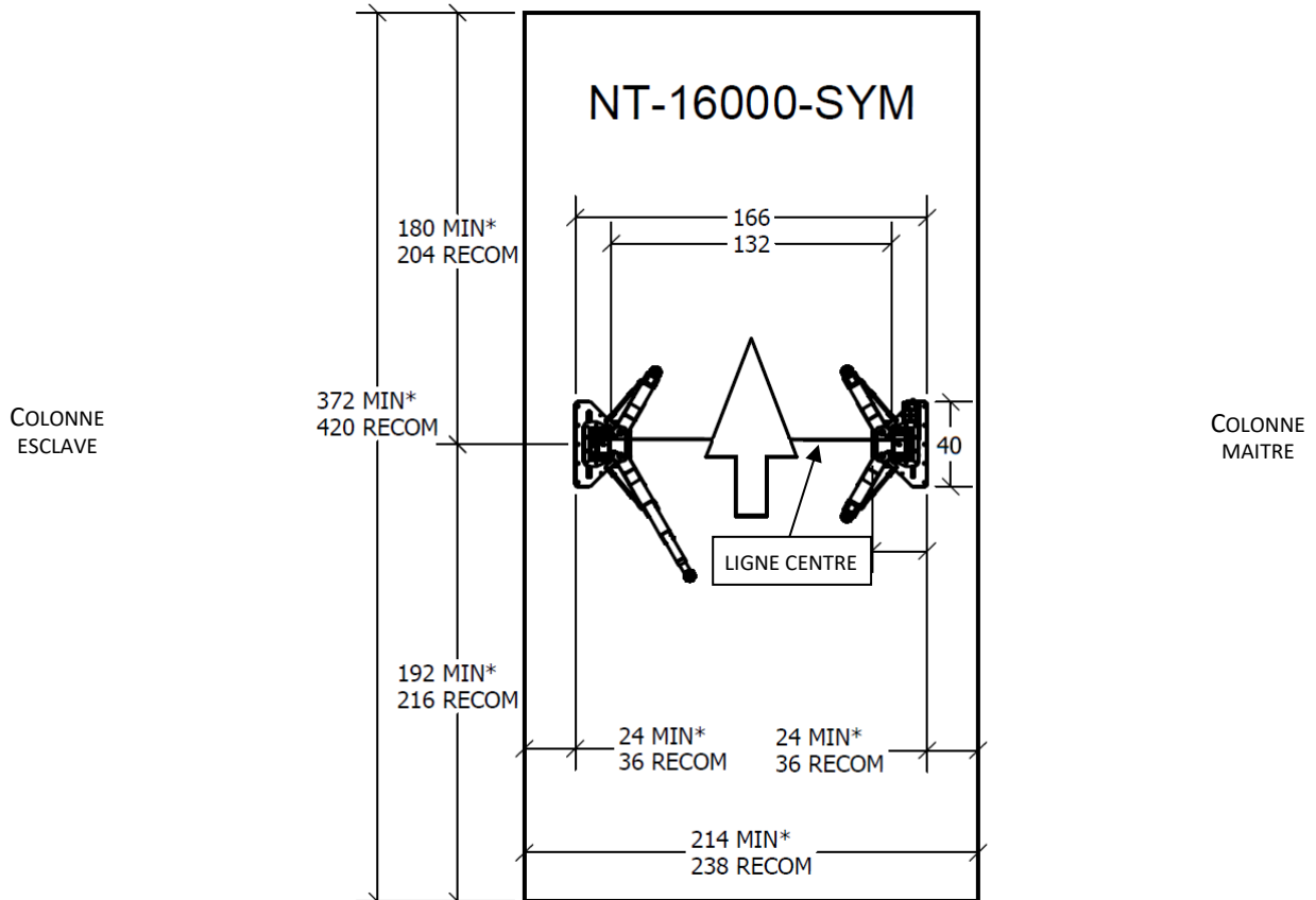
FIGURE 5 : DIMENSIONS DE LA BAIÉ DE TRAVAIL MINIMALES ET RECOMMANDÉES
