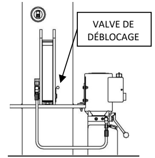
FIGURE 13 : VALVE DE DÉBLOCAGE
