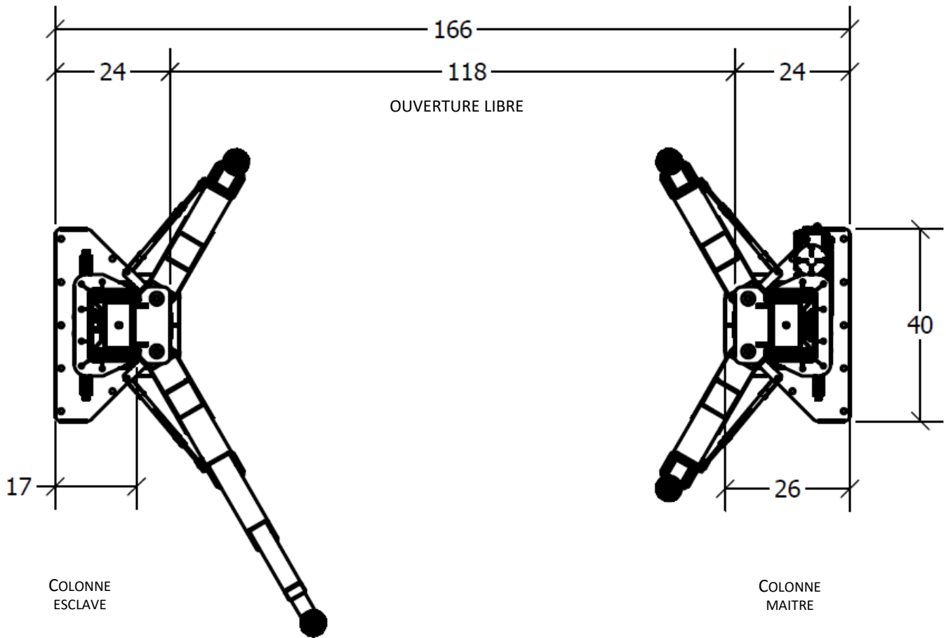
FIGURE 3 : VUE AU-DESSUS DU PONT ÉLÉVATEUR
