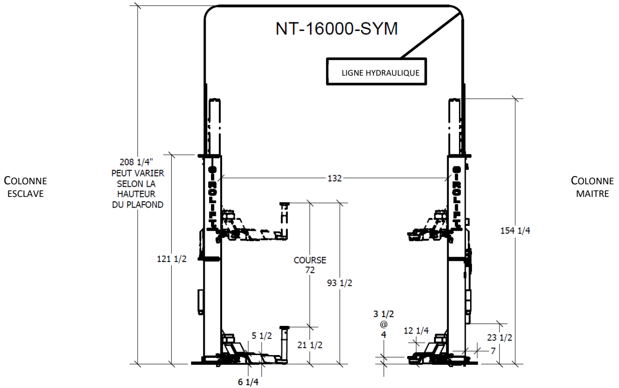
FIGURE 4: VUE LATÉRALE DU PONT ÉLÉVATEUR
